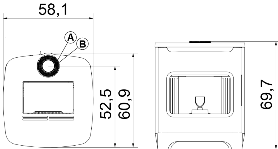
Fig. 14 - Allmänna mått: FLOS 6
