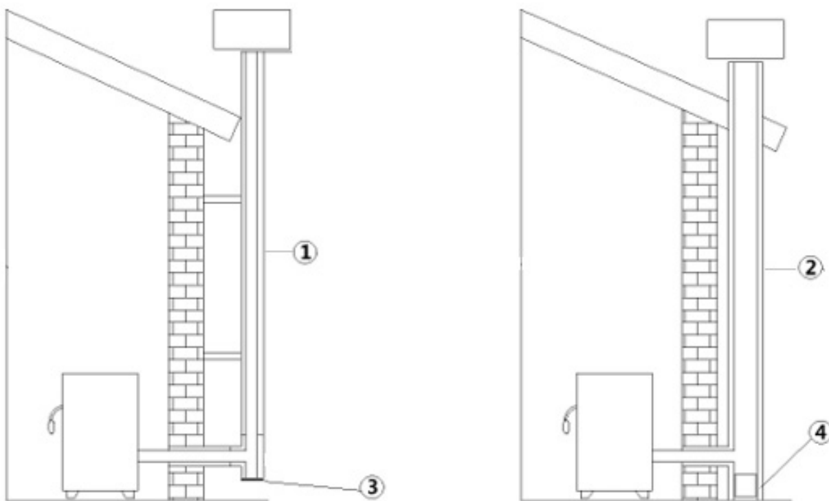
Fig. 3 - Skorstensrör
