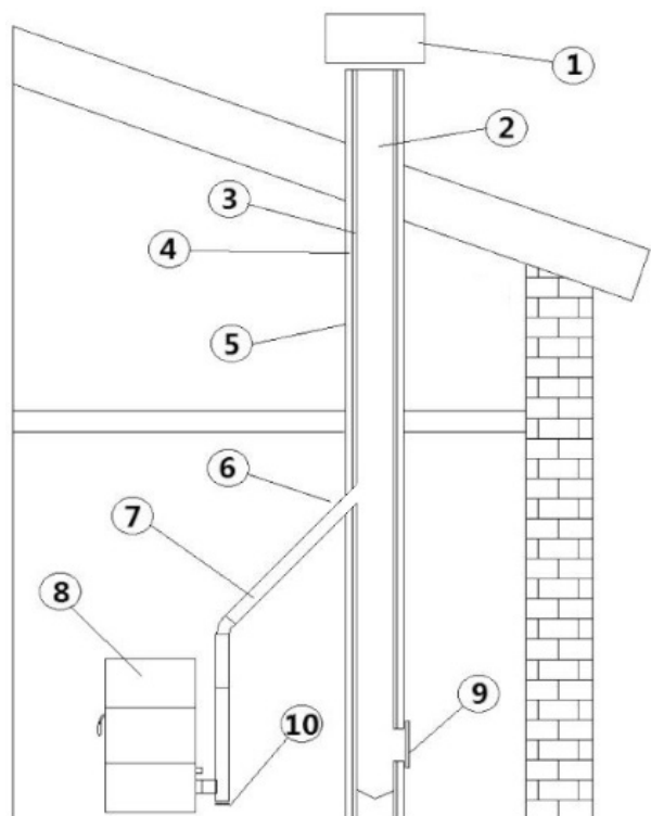
Fig. 2 - Skorstenens komponenter
