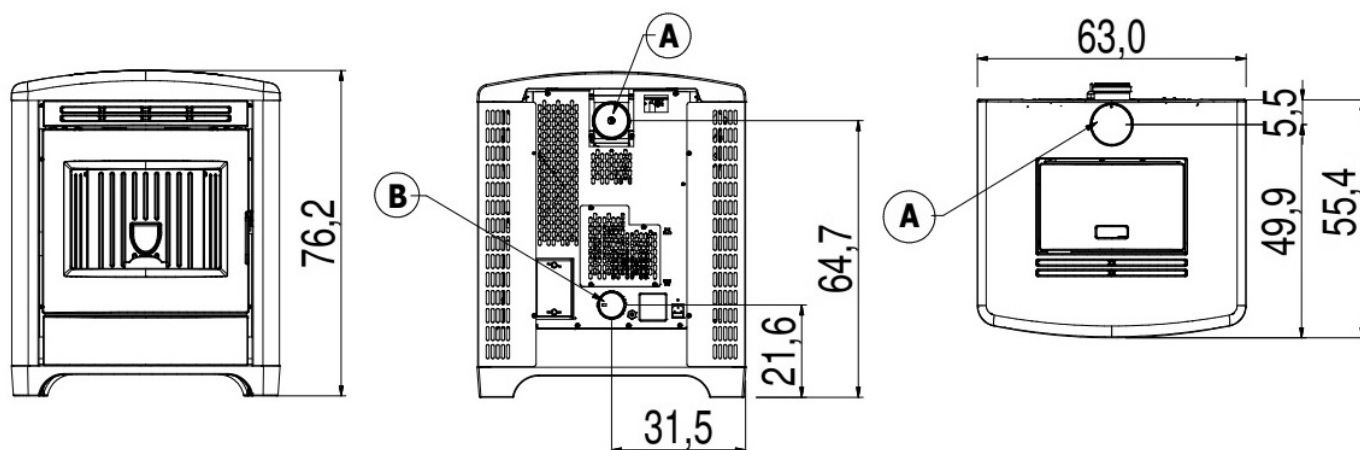
Fig. 12 - Allmänna mått: MAGRITTE 6
