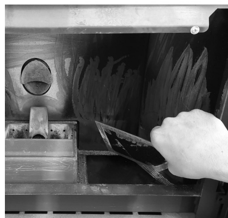
Fig. 25 - Ta bort inspektionslocket
