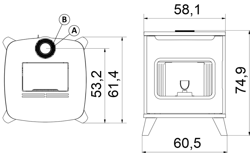
Fig. 13 - Allmänna mått: HUBLLOT 6 UP
