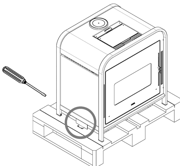
Fig. 1 - Borttagning av fästen
